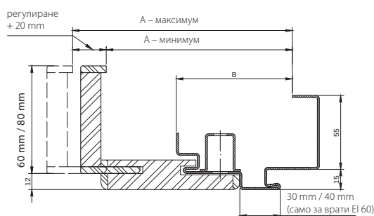
разрез на каса ПРОЕКТ
