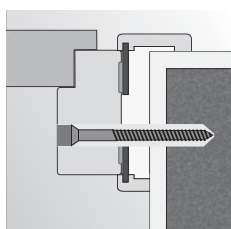
монтаж с пяна и анкер към стена
