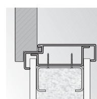
голяма Ъглова каса монтаж върху стена от гипскартон
