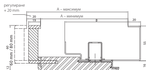
разрез на каса ПРОЕКТ Премиум
