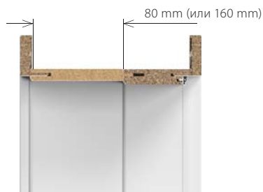
вариант с регулиращ панел (80, 160 mm)
