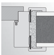
монтаж с пяна към стена
