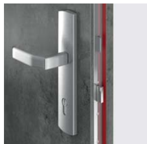
езична многоточкова брава Winkhaus, тип кука-болт
