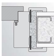
монтаж с пяна към гипсокартон
