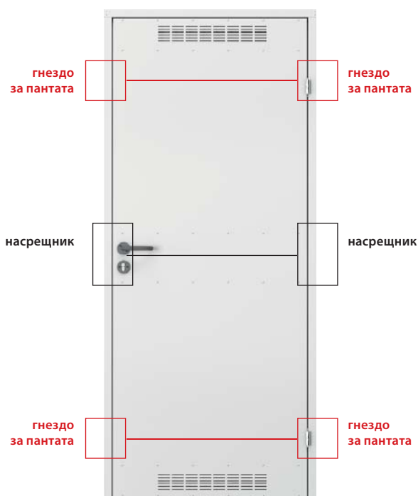
изглед на крилото отпред
