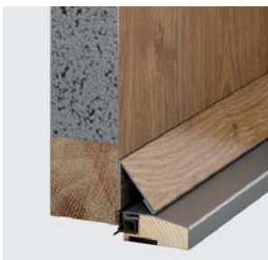
Пълнеж - експандиран пенополистирол
