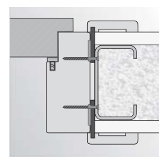
монтаж с дюбели към гипсокартон
