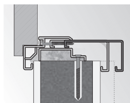
каса Регулируема
