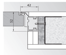
Със срещуположен фалц (отваряне навътре)
