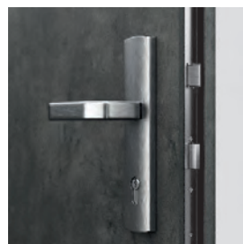
лентова многоточкова брава Winkhaus, със куковидно-езично заклучване
