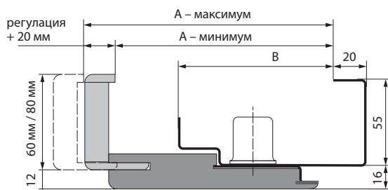
напречно сечение на каса ПРОЕКТ Премиум
