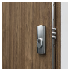
патронна лентова брава с многоточково шиповидно заключване, пригодена за две секретни ключалки
