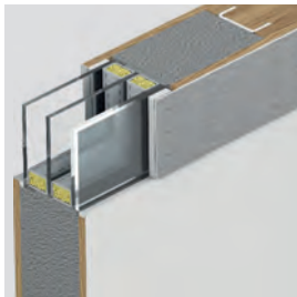
двакамерен стъклопакет, клас на противовзломност P4, рамкиран с неръждаема стомана
