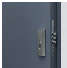
Врата Стийл СЕЙФ - тип II Горна брава - секретна с три шипа
