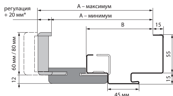
напречно сечение на каса ПРОЕКТ БИС
